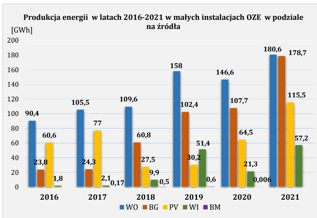
Rysunek 2. Produkcja energii w małych instalacjach OZE w latach 2016-2021 w podziale na rodzaj źródła (w GWh)
